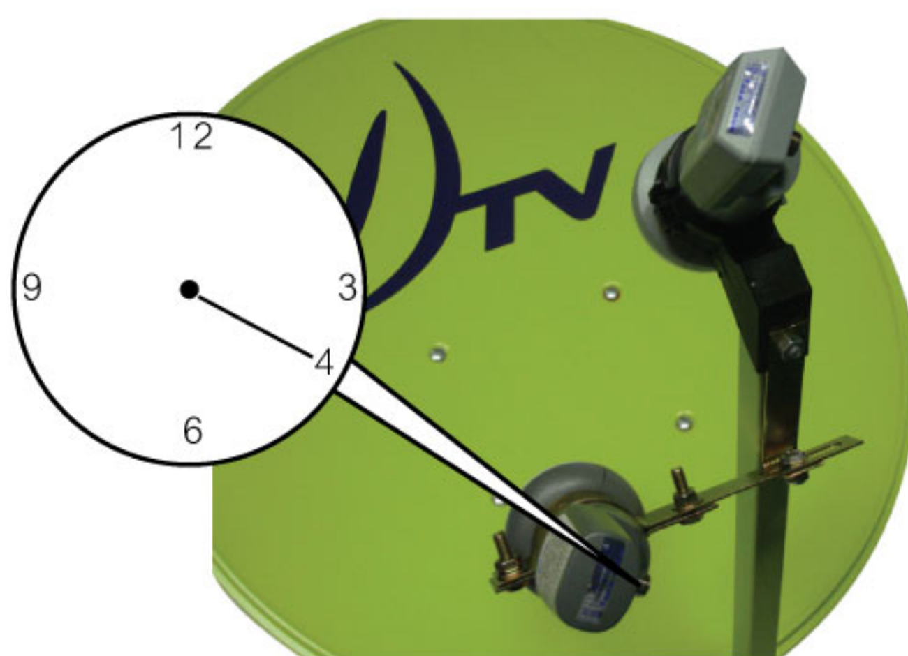
ประกอบหัวรับ LNB K1U หัน F-TYPE ของ LNB มาทาง 4 นาฬิกา
