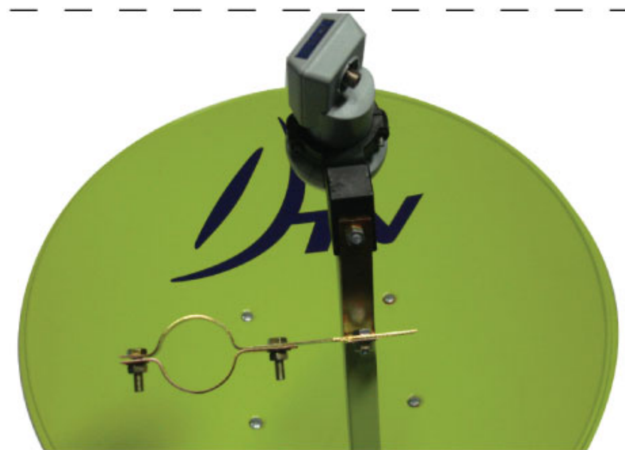
ประกอบขาจับ LNB เรียบร้อยแล้ว
